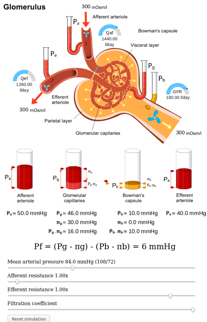
Obrázek 4 – Simulátor glomerulu (anglická verze). Simulátor je realizován jako interaktivní obrázek propojený se simulačním modelem v pozadí. Bowmanovo pouzdro (oranžově), aferentní a eferentní arterioly. Červené šipky symbolizují směr proudění krve, žlutá šipka ukazuje směr proudění moči. Pro každou část glomerulu se vypočítá jak hydrostatický, tak i osmotický tlak. Rozdíl mezi celkovým efektivním tlakem v kapilárách a v Bowmanově pouzdře (vizualizovaný válci) řídí čistý filtrační tok. Uživatel může měnit střední arteriální tlak, rezistence v aferentní a eferentní arteriole a filtrační koeficient. Následně může pozorovat důsledky těchto změn. Ve výukové aplikaci je simulátor doprovázen vysvětlujícím textem.
