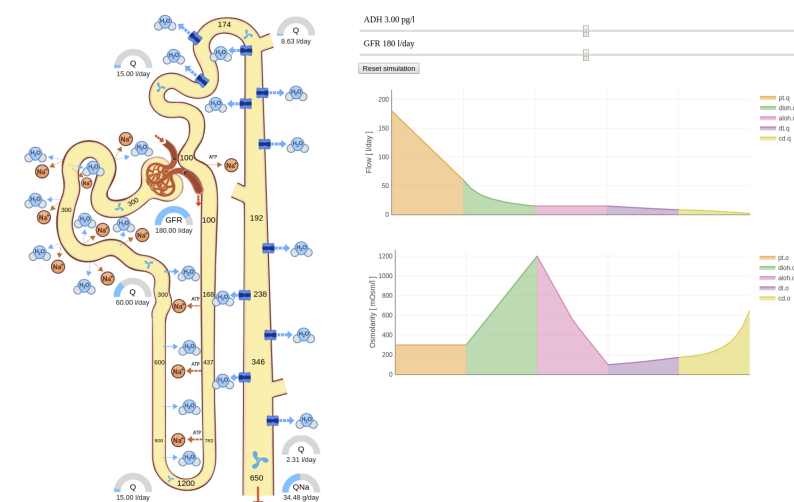
Obrázek 5 – Jeden z interaktivních obrázků anglické verze webového simulátoru ledvin, zobrazující nefron jako celek – v jednotlivých částech nefronu jsou zobrazeny hodnoty osmolarit a průtoků. V grafu se zobrazuje tok a osmolarita v jednotlivých částech nefronu. Obrázek je propojen s modelem na pozadí. Uživatel může na tomto interaktivním obrázku změnit hladinu ADH a glomerulární filtraci a pozorovat důsledky této změny.
